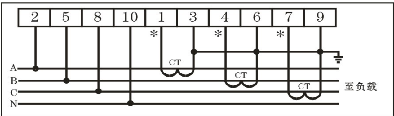
三相四线，电流互感式（电压 3 \times 220/380\text{V} ，电流 3 \times 1.5 （ 6 ）A）；*号端，为电流进线端
