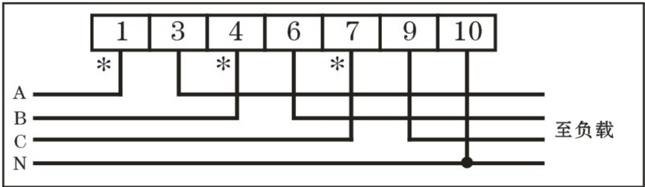
三相四线，直接式（电压 3 \times 220/380\text{V} ，电流 \geq 3 \times 5 （ 20 ）A）；*号端，为进线端
